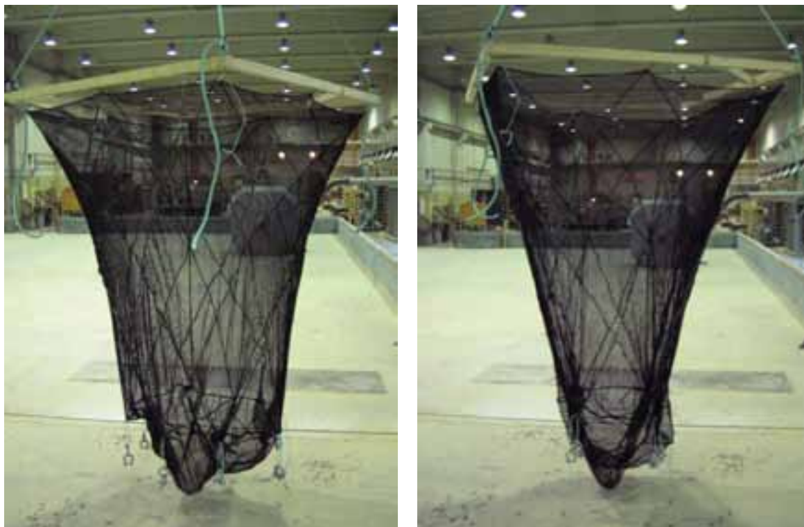
Figur 14: Not 5 uten sidetau i hjørnene. Venstre: Sidetauene er fjernet. Høyre: Notlinfelt i bunnen er stripset sammen i et forsøk på å unngå poser.
