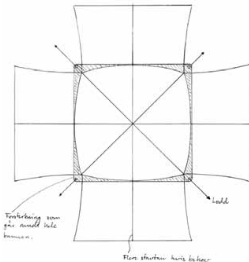
figur 2 – Siden nota oftest ryker i overgang mellom side og bunn, bør man gi dette området spesiell oppmerksomhet. En “rammekonstruksjon” av fiberforsterket materiale (dvs som ikke tøyer seg) rundt hele denne kanten, kan muligens gi ekstra styrke her.
