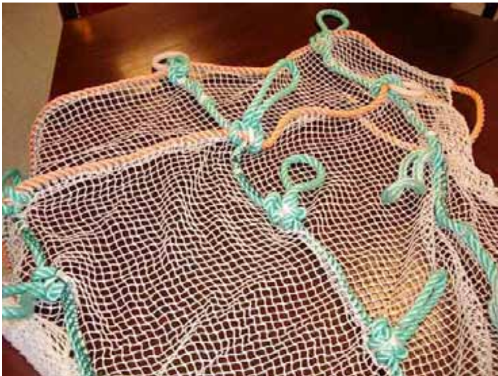
Bilde 1: Modell av notpose (side). Grønne tau er vertikale stavtau. Øverste røde tau er toppen av "hoppnett". Neste røde tau er topptau, med grønne løkker som fester noten til flyteren. Man ser at notlinet blir sydd direkte fast (gjennom) tauverket (reduserer slitasje).
