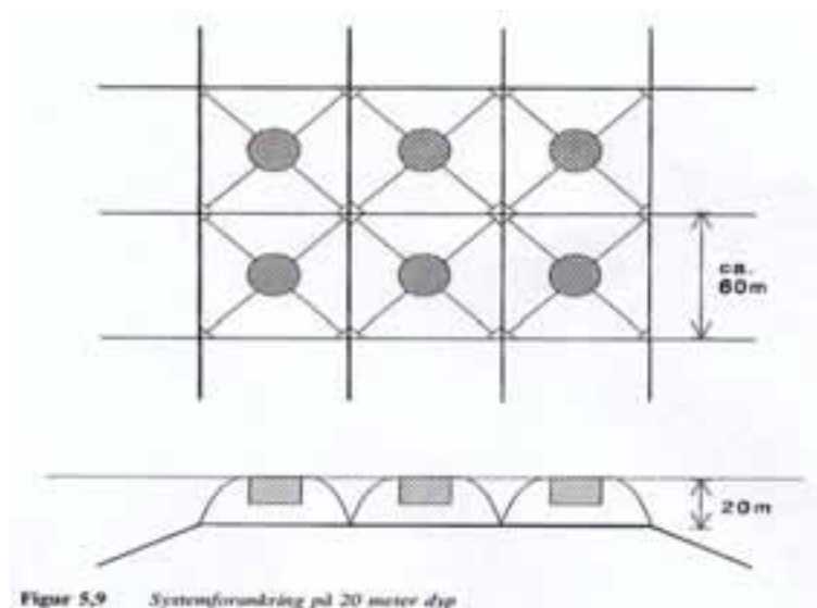
Figur 4.2. Systemforankring med senket ramme. Gir horisontal fleksibilitet.
