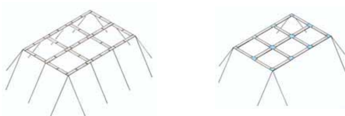
Figur 4.1. Sammenheng mellom antallet liner (dagens praksis til venstre, reduserte liner til høyre) og strukturmessig krav. Horisontal fleksibilitet må tas opp på en annen måte når antallet liner reduseres.
